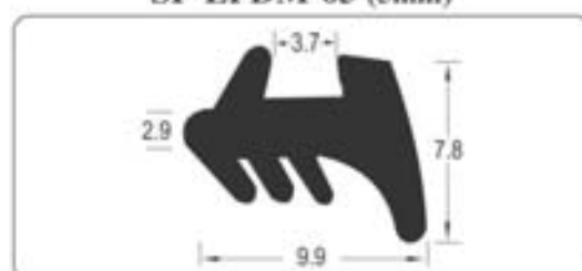
SP-EPDM-05 (5mm)
