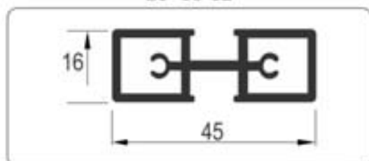
SP-16-12
