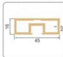
SP-16-11 MG
