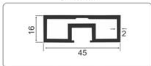
SP-16-11
