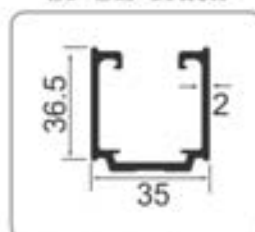
SP-SL-Track
