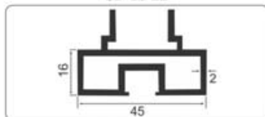
SP-16-22
